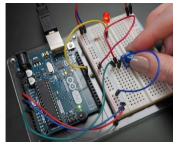
Circuito Arduino
