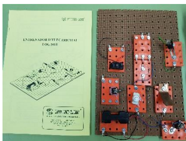
Entrenador de electricidad
